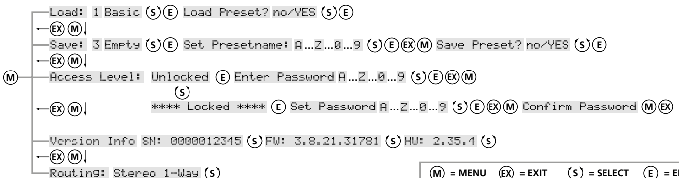
Abb. 7 Menüstruktur des Systemmenüs
